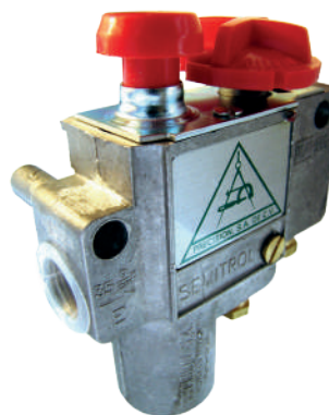
TERMOSTATO SEMIAUTOMÁTICO
